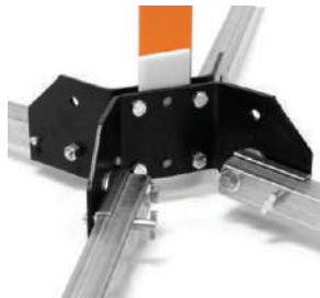
T-Pin*
